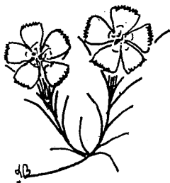
Garofano dei Ghiacciai.
