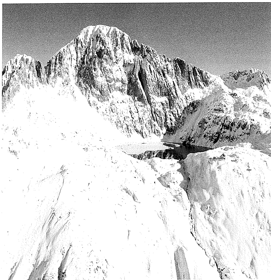
Foto 1. Cima d'Asta con il suo lago e la soglia in roccia formati dall'azione erosiva del ghiacciaio.
