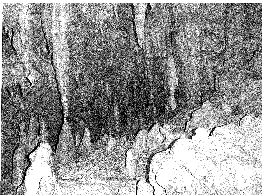
Foto 7. Stallatiti e stalagmiti nella Grotta di Castel Tesino.
