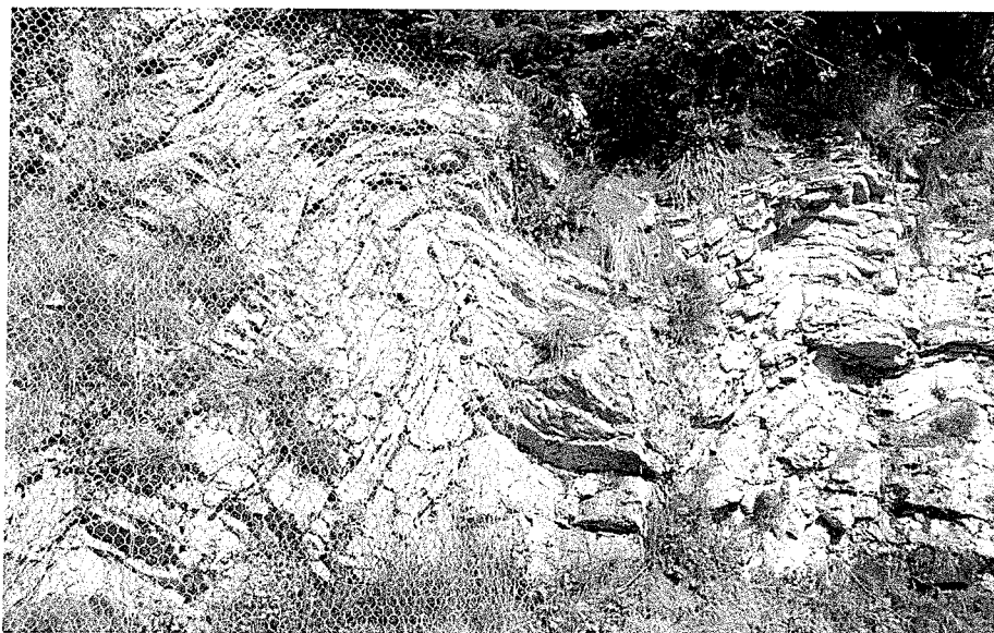
Foto 4. Pieghe nella formazione rocciosa della Scaglia Rossa.
