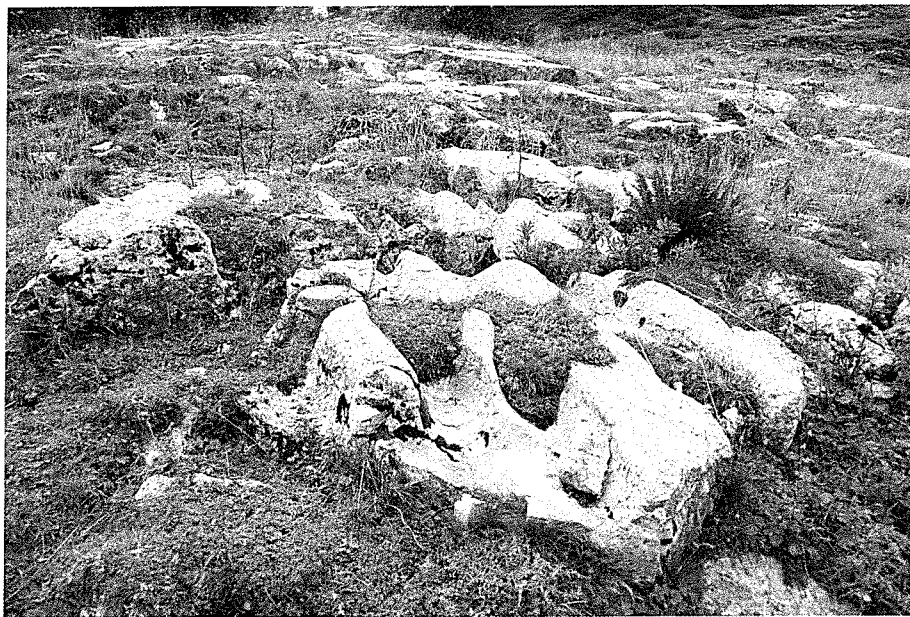
Foto 8. Scannellature carsiche arrotondate.
